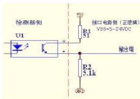
图 7-正逻辑接法
