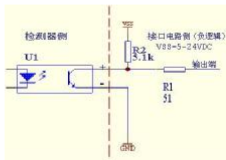
图 8-负逻辑接法
