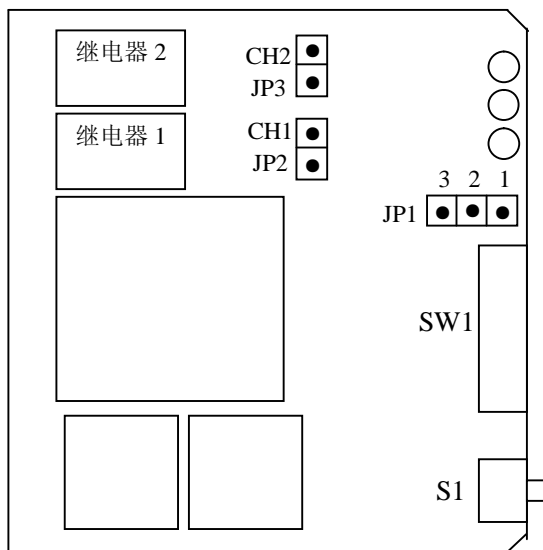
图 2 (主板示意图)
